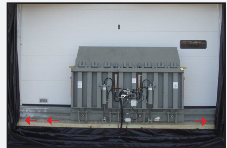
El conjunto de carro de rodillos permite el movimiento lateral para adaptarse a la posición del vagón.
